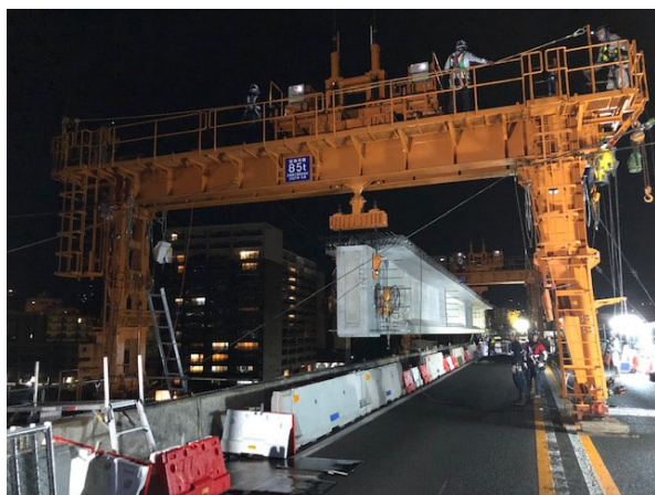
＜橋梁桁架設＞
