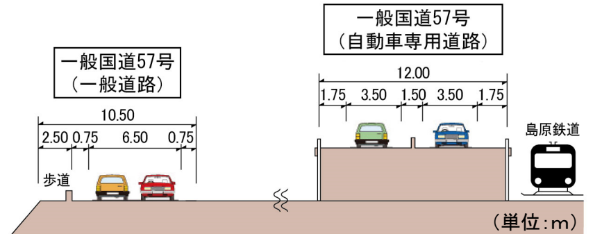
<今回開通区間の標準横断面図>
