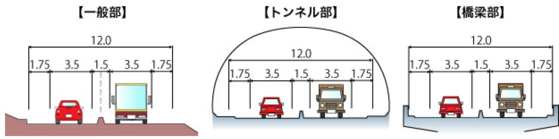
＜今回開通区間の標準横断面図＞
