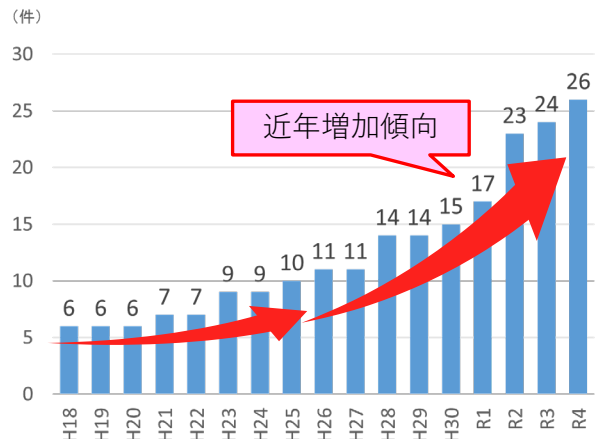
▲国道204号通行規制の累計
