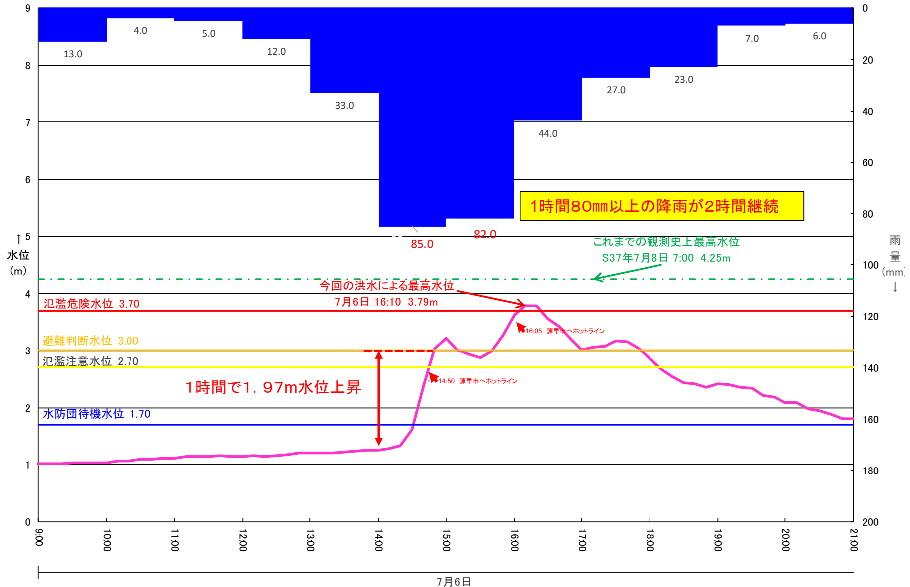
本明川水系本明川 令和2年7月6日出水 裏山水位観測所—小野雨量観測所
