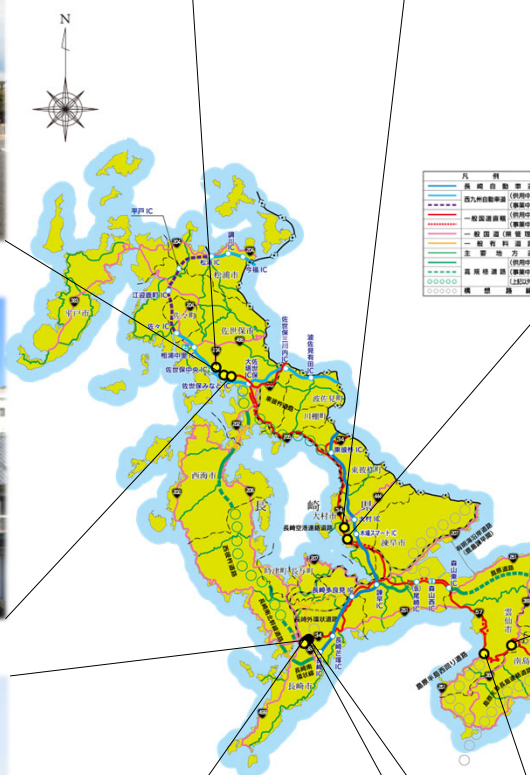
国道34号 玖島地区電線共同溝 2.08 km(道路延長1.04km)
