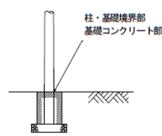
基礎コンクリートが露出している場合
