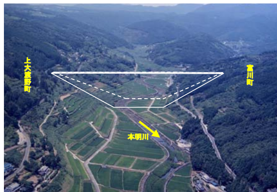
写真5-1-1 本明川ダムサイト予定地
