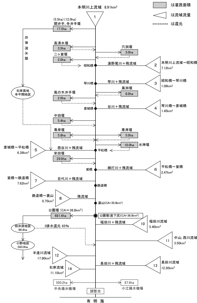
図2-2-1 本明川取排水系統図
