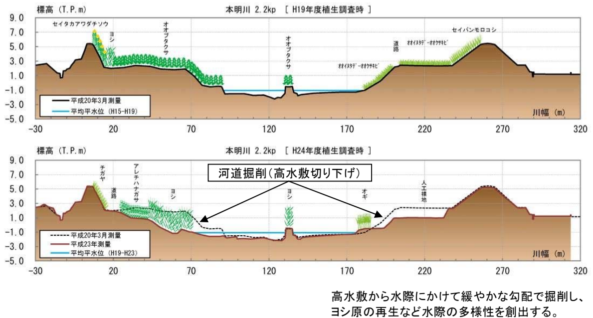
図5-1-6 河道掘削による横断形状の変化イメージ
