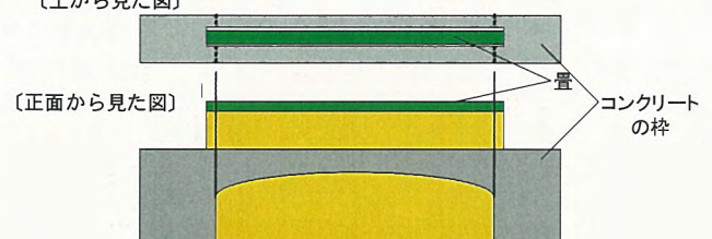
図 1-2-2 畳堤詳細図
