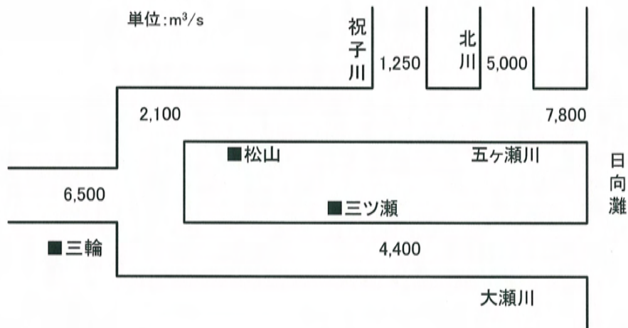
図 3-4-1 流量配分図
