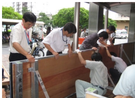
止水板設置訓練実施状況(宮崎県立病院)
