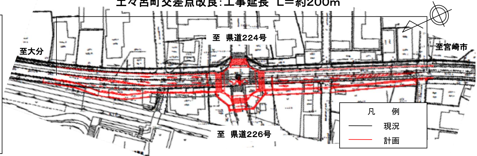
土々呂町交差点改良:工事延長 L=約200m
