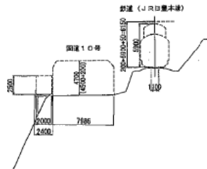
設計条件(河川部)
