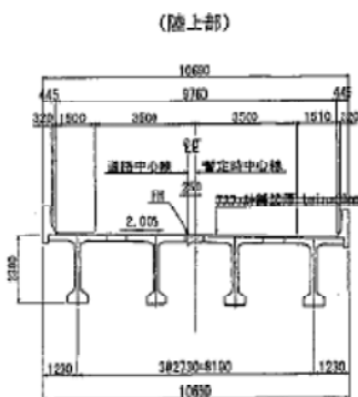
設計条件(陸上部)
