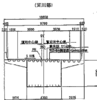
上部工標準断面図 S=1:100
