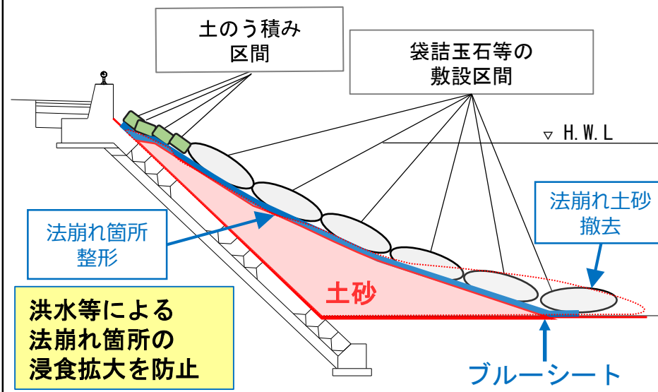
今回の応急復旧の施工断面イメージ
