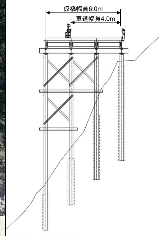
仮橋部断面図
