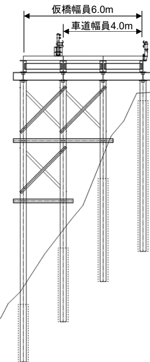
仮橋部断面図
