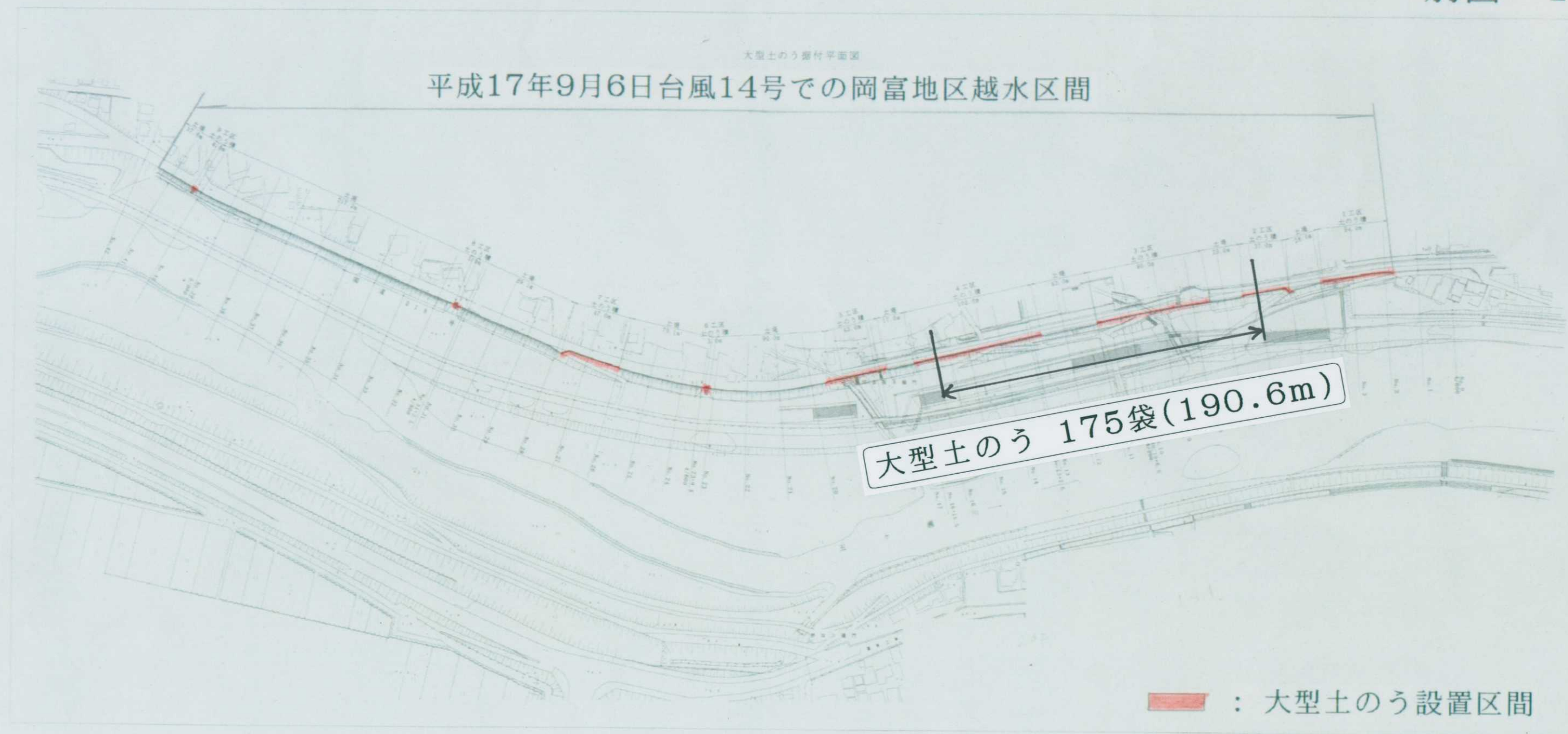
図 1-1 大型土のう据付平面図
