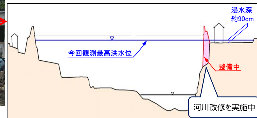
〈大野川 上戸次地区横断面イメージ〉
