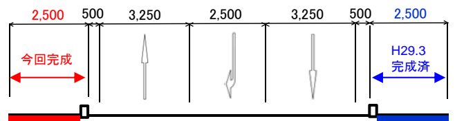
整備後 (A-A)
