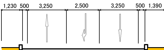
整備前 (A-A)
