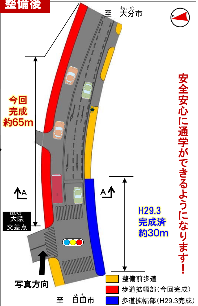
整備後 (A-A)
