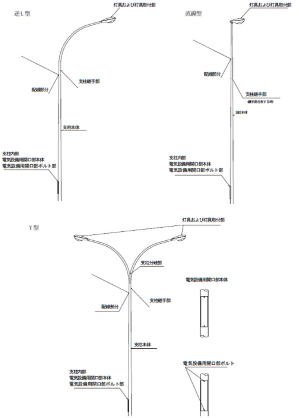
付図-1-2 主な点検箇所（ポール照明方式）
