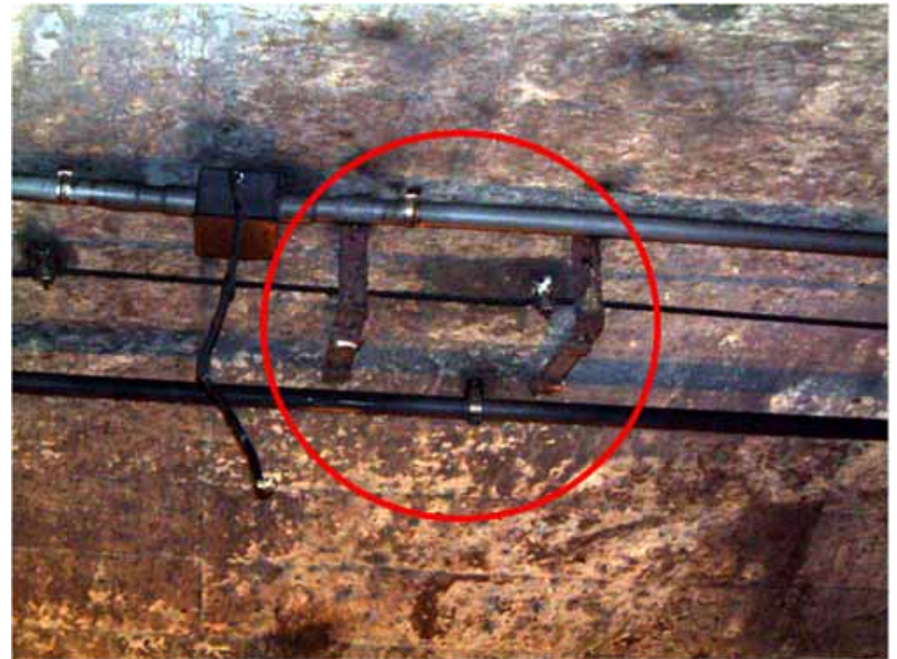
落下後の照明取付け部
