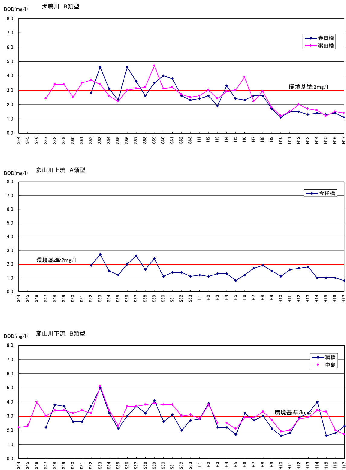
図2.2.3 (2) 遠賀川水系におけるBOD75%値の経年変化図 (2/3)
