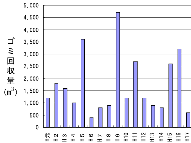
図2.2.6 遠賀川河口堰におけるゴミ回収量
