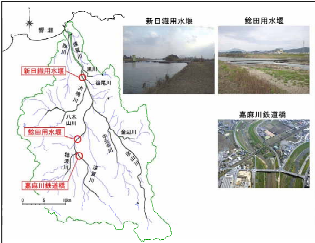
図2.1.2 主な洪水流下阻害の横断工作物
