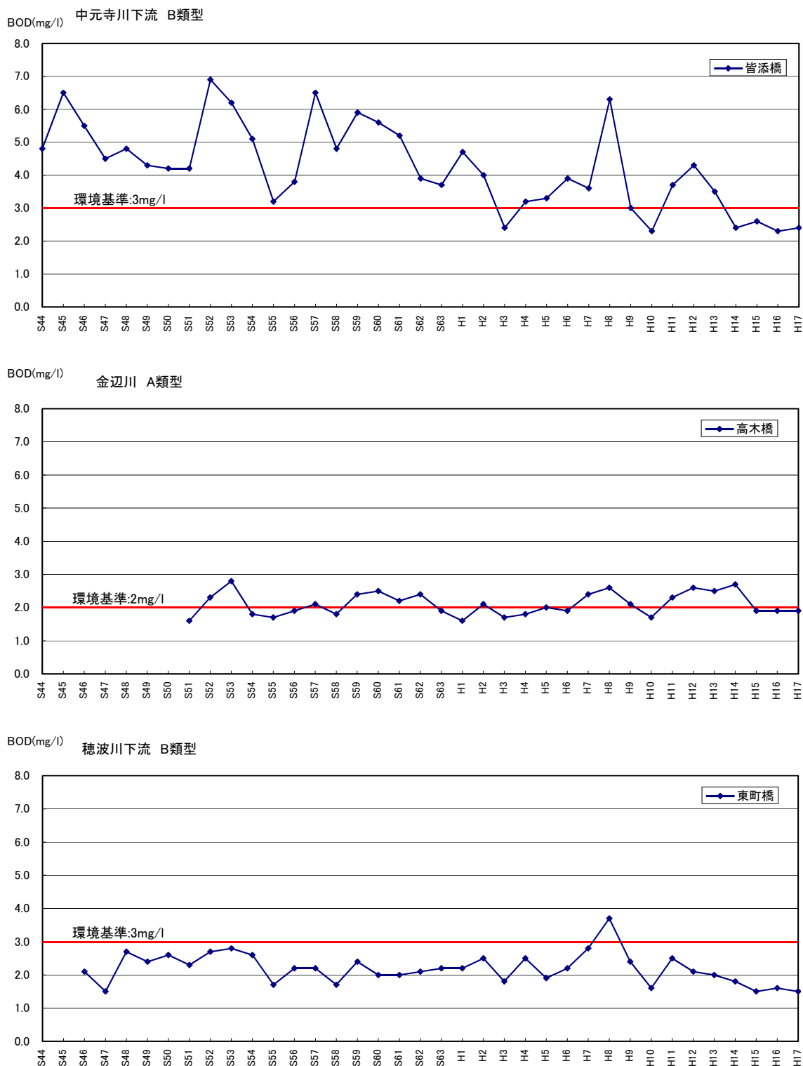
図2.2.3 (3) 遠賀川水系におけるBOD75%値の経年変化図 (3/3)
