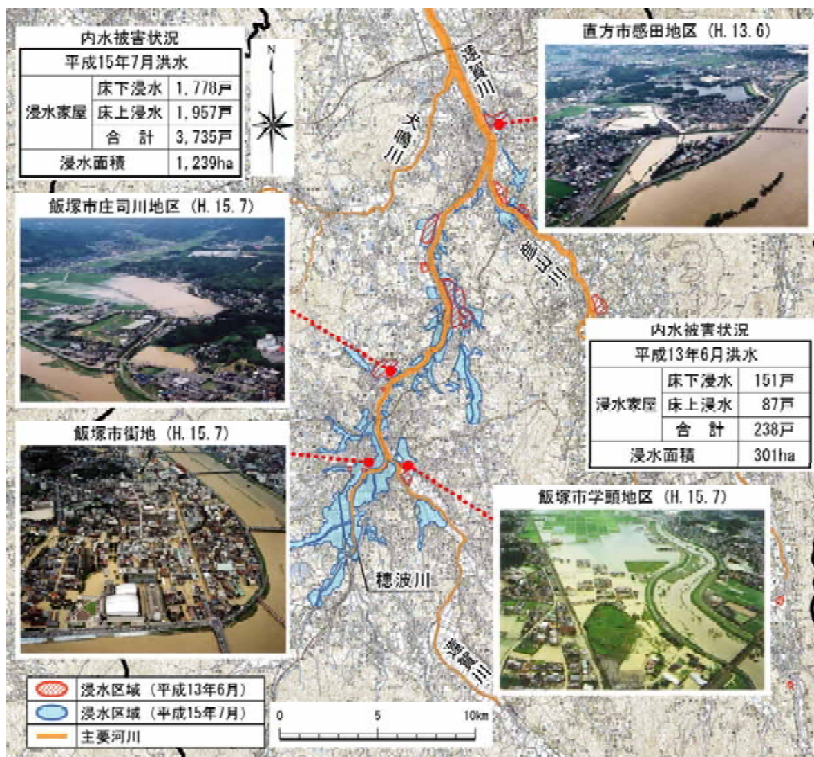
図2. 1. 4 近年の内水被害状況図（平成13年6月、平成15年7月）
