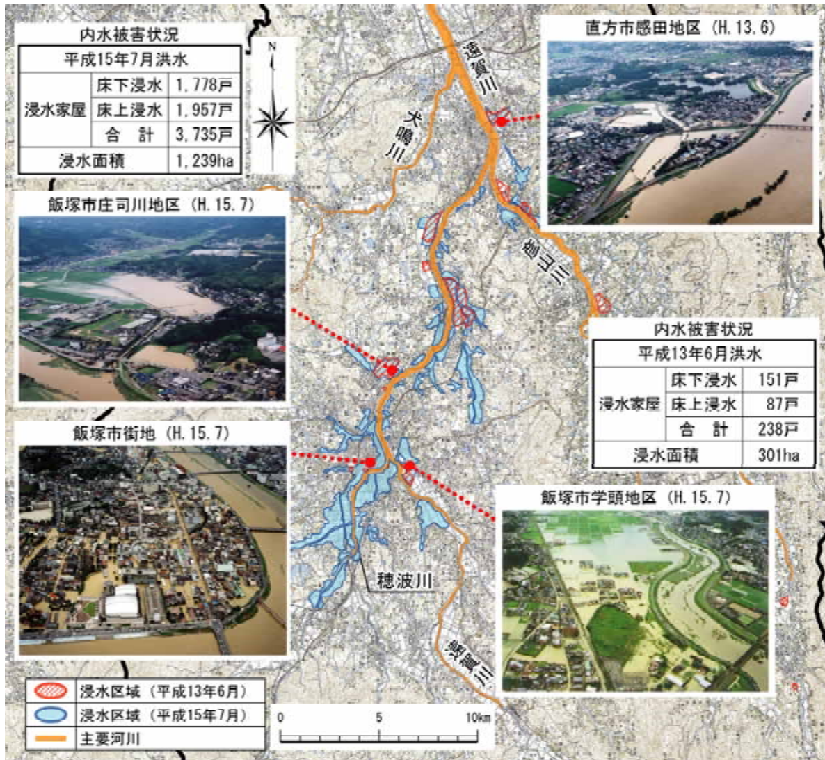
図2.1.4 近年の内水被害状況図（平成13年6月、平成15年7月）
