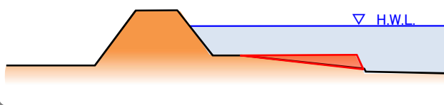
掘削イメージ
