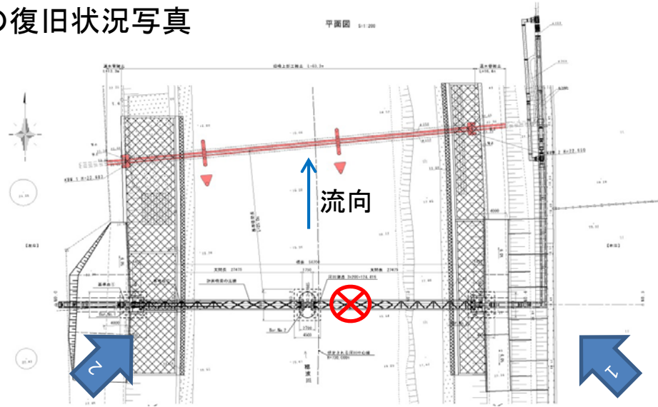
旧橋撤去平面図
