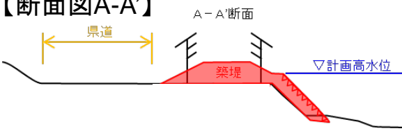
【断面図A-A'】
