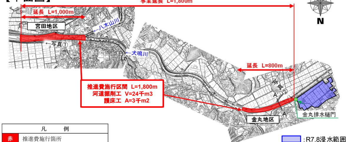
【平面図】
