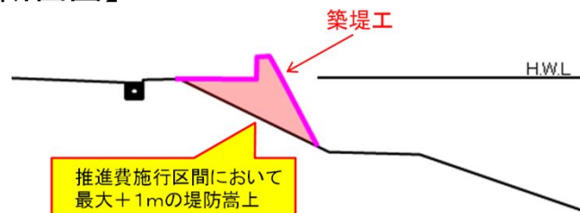
【断面図】
