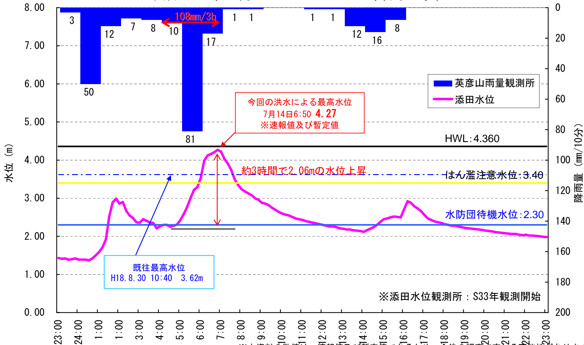
平成24年7月13日～14日の降雨と水位
