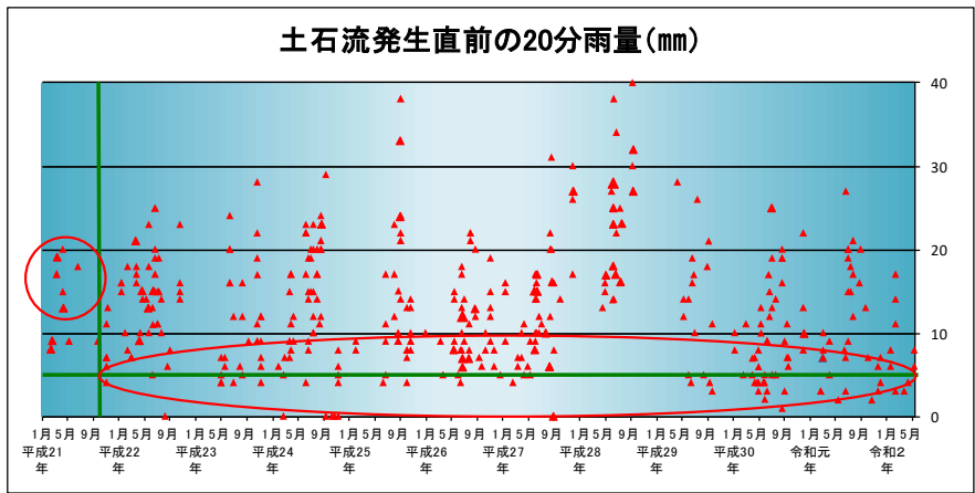
土石流発生直前の降水量(平成21年3月1日～令和2年5月31日)
