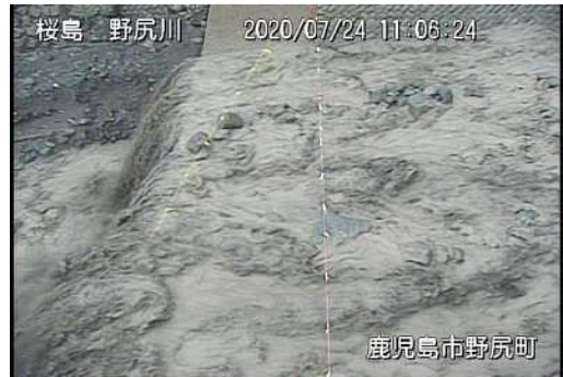
野尻川土石流の様子(7月24日)
