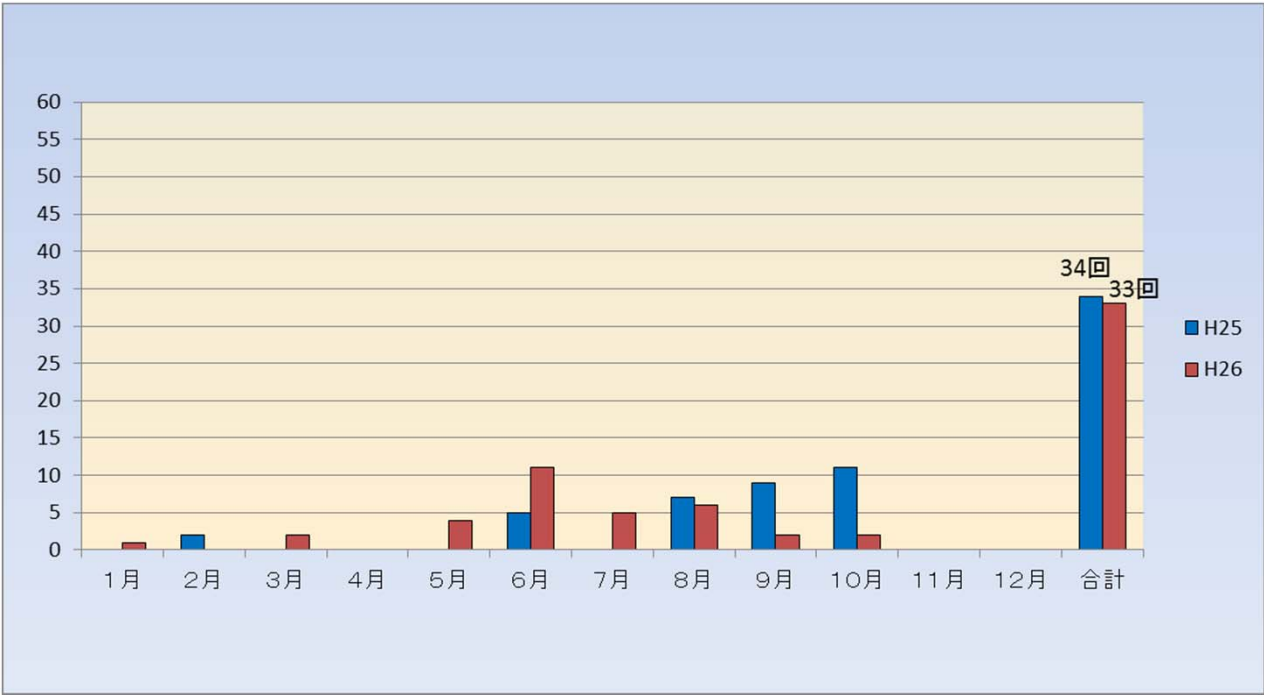
2013年及び2014年(1月～10月)の土石流発生回数比較
