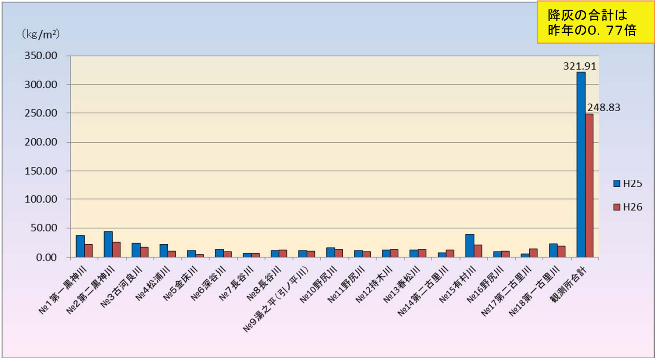
2013年(1～9月)及び2014年(1～9月)の降灰量比較
