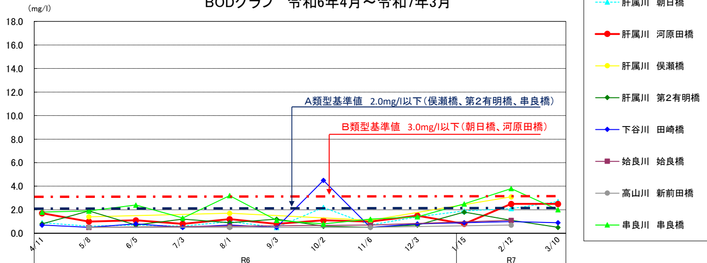
BODグラフ 令和6年4月～令和7年3月
