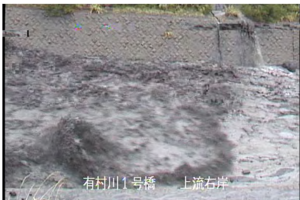
有村川 土石流の様子(11月 1日)
