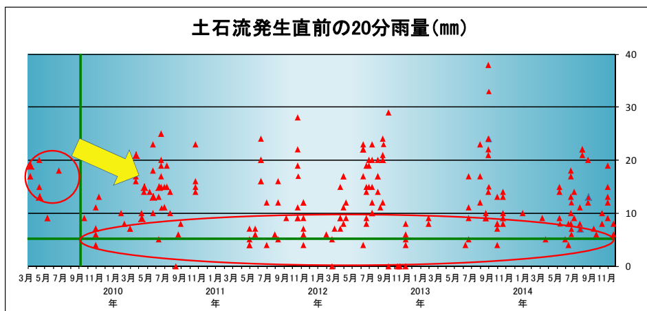
土石流発生直前の降水量(2009年3月1日～2014年11月30日)
