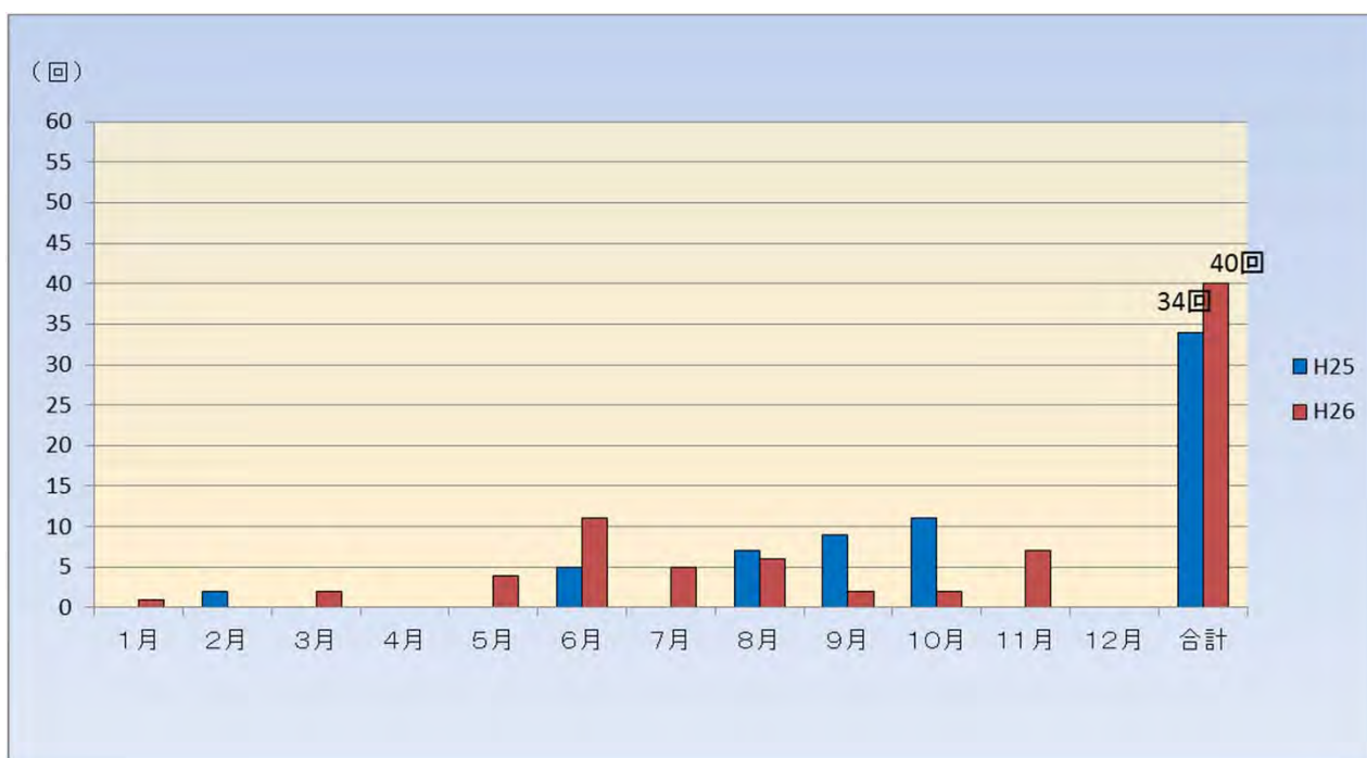
2013年及び2014年(1月～11月)の土石流発生回数比較
