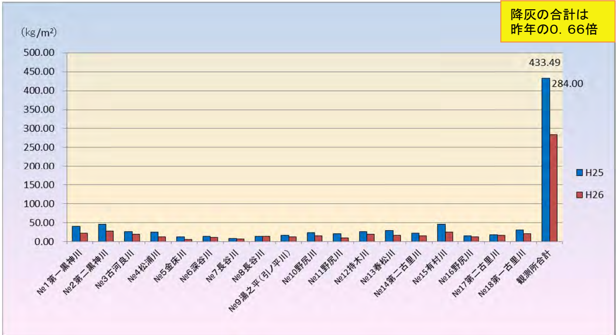
2013年(1~10月)及び2014年(1~10月)の降灰量比較
