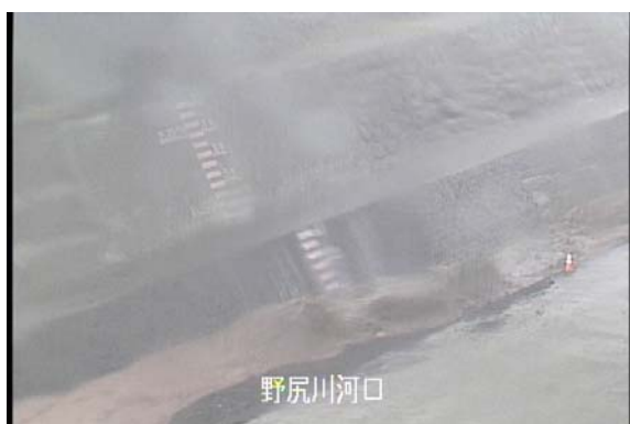
野尻川 土石流の様子(7月20日)
