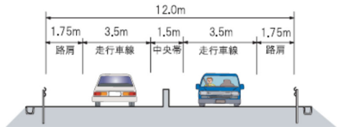
土工部
