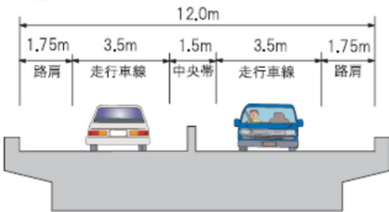
橋梁部
