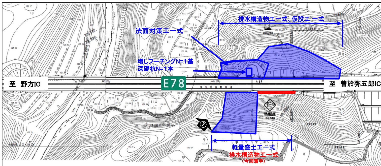
【復旧平面図】
