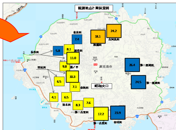
桜島の降灰観測結果(2015年1月～12月)累計
