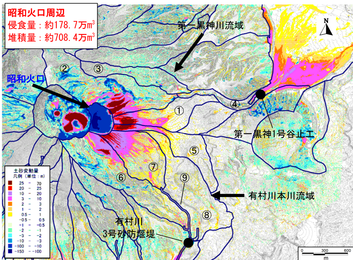
参考図7 昭和火口周辺侵食堆積図（平成18年11月～平成27年11月）
