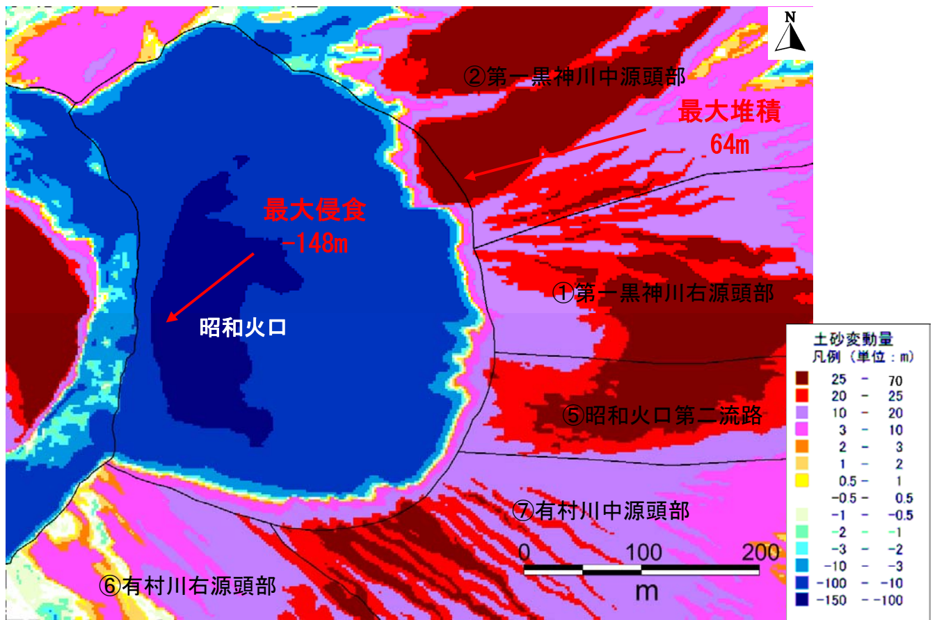
参考図6 昭和火口周辺最大侵食・堆積状況図 (平成18年11月～平成27年11月)
