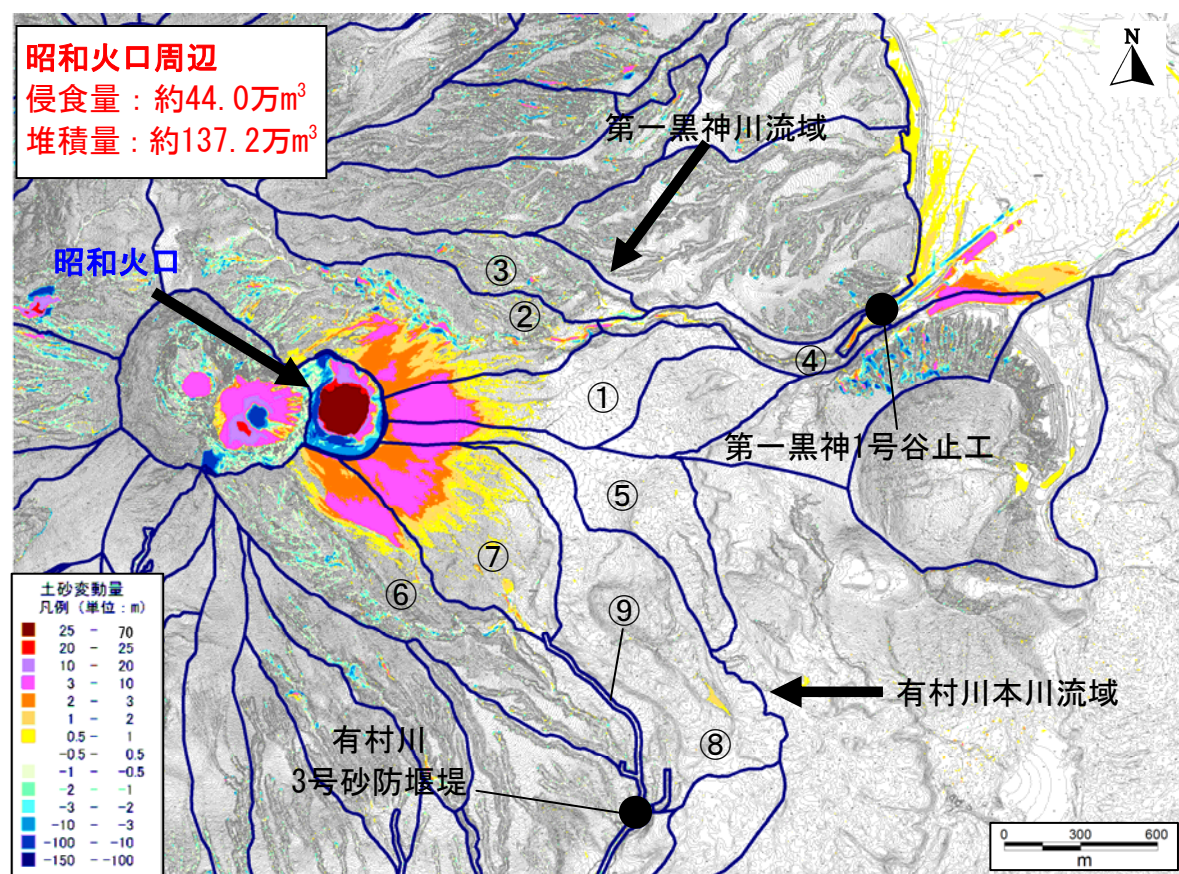
図4 昭和火口周辺侵食堆積図（平成26年10月～平成27年11月）
