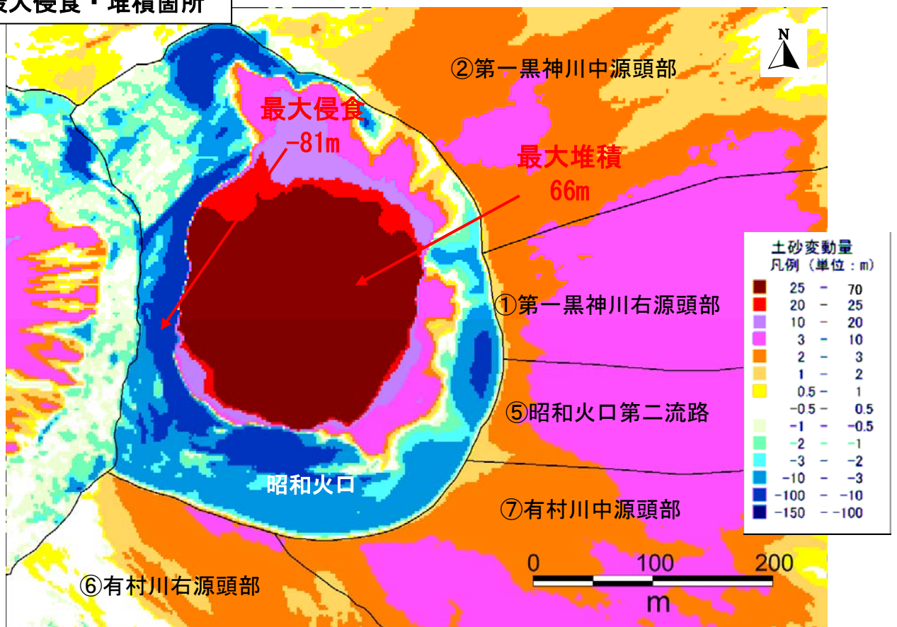
図3 昭如火口周辺最大侵食・堆積状況図 (平成26年10月～平成27年11月)
