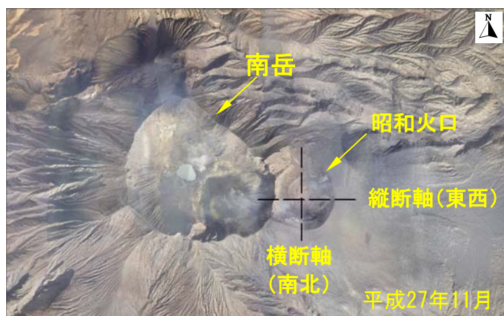
図1 昭和火口形状の経年変化位置図
