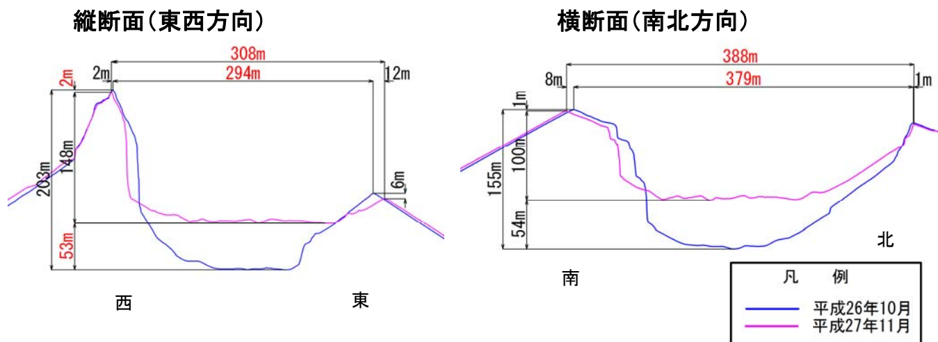
図2 昭和火口形状の経年変化（平成26年10月～平成27年11月）
