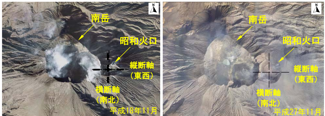
参考図1 昭和火口形状の経年変化位置図（平成18年11月，平成27年11月）
