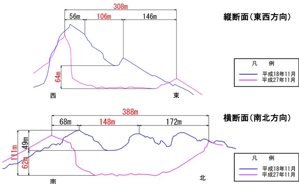
参考図2 昭和火口形状の経年変化（平成18年11月～平成27年11月）
