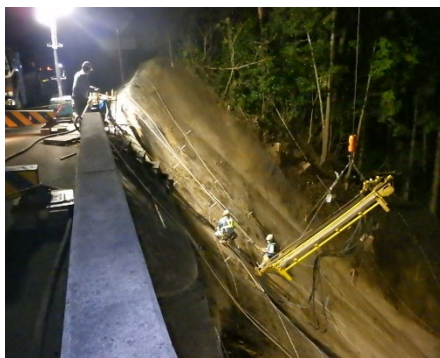
法面の補修
