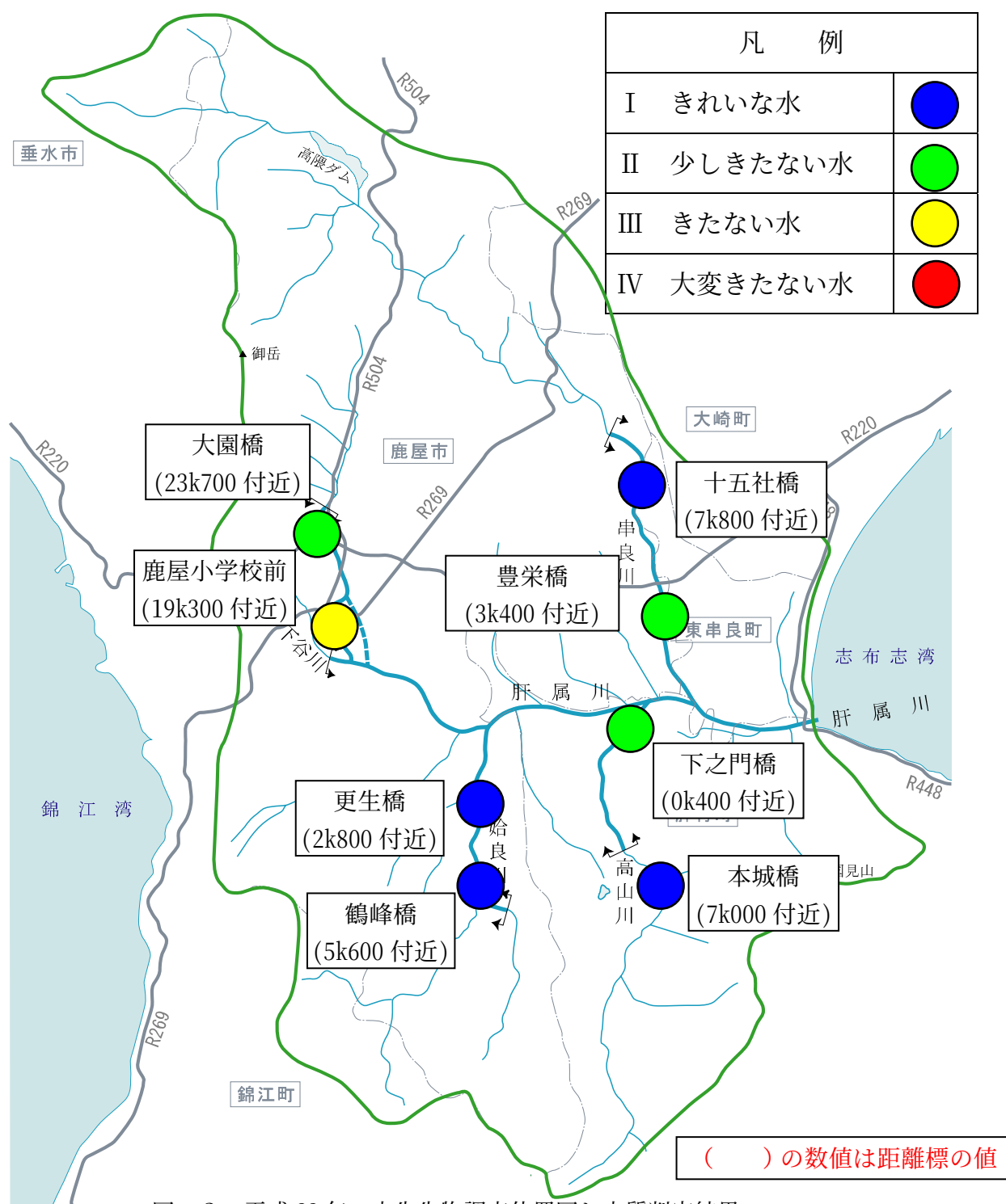
図－3 平成 22 年の水生生物調査位置図と水質判定結果
