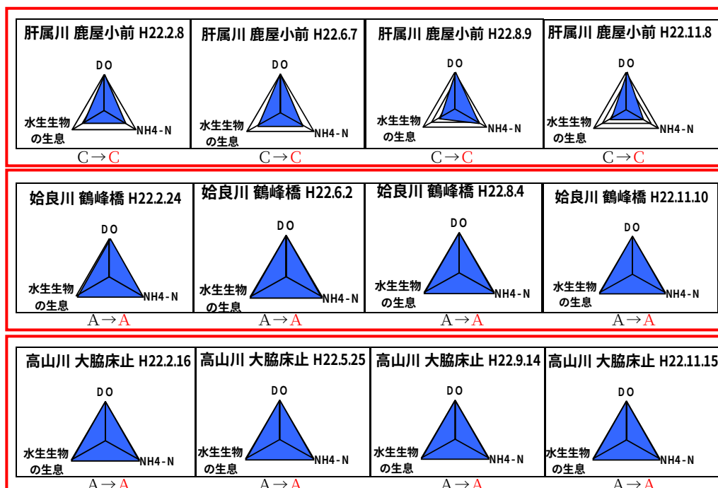
図ー5 平成22年「豊かな生態系の確保」調査結果
