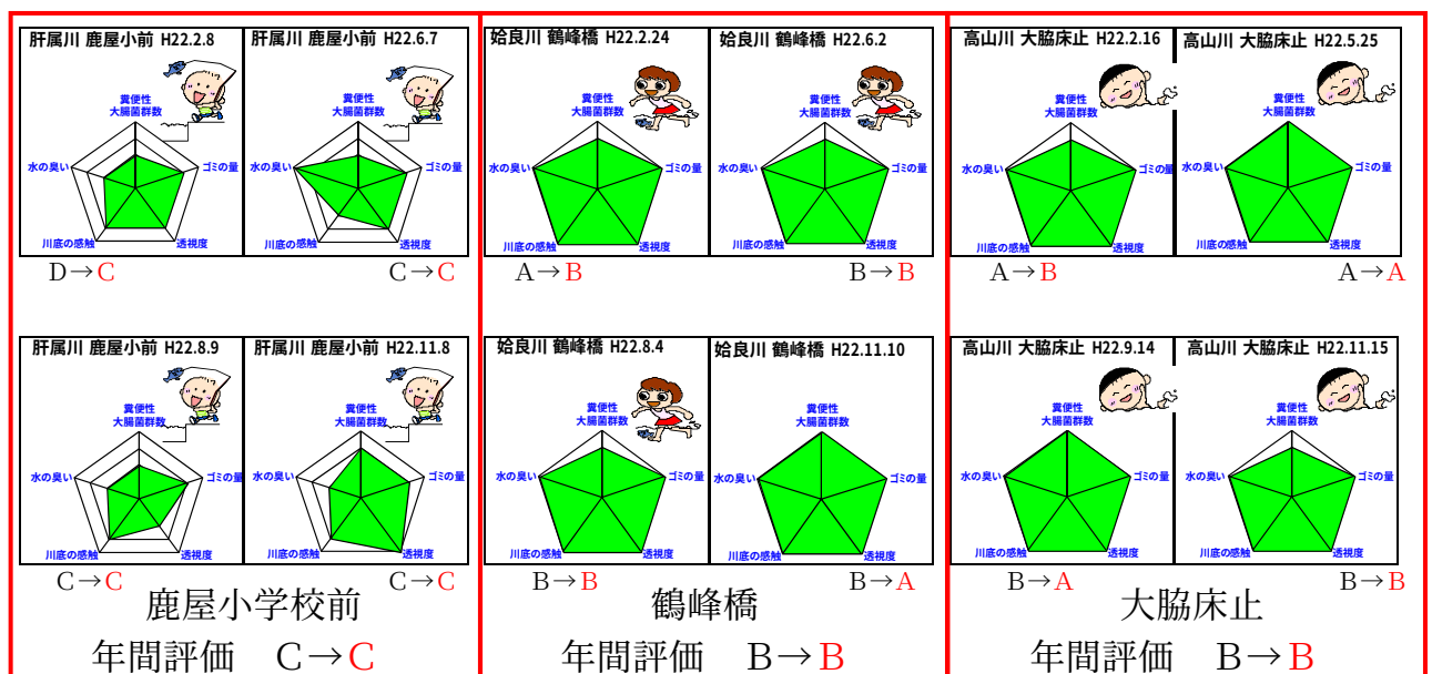
図－4 平成22年「人と河川の豊かなふれあいの確保」調査結果
