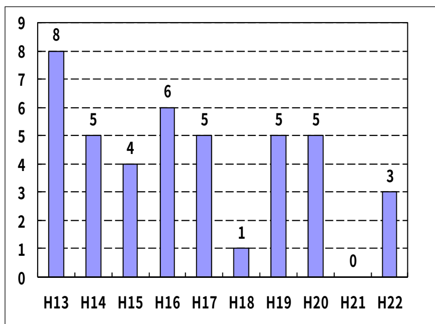
図－6 水質事故発生件数の経年変化
