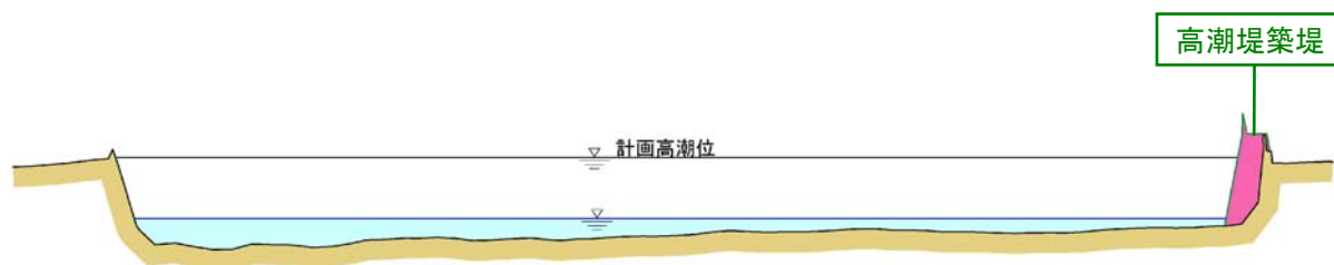
図 4.2.23 高潮対策イメージ図 (肝属川本川 0k 400 付近)
