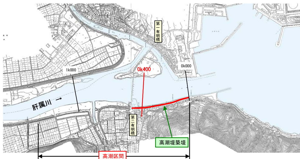
図 4.2.22 高潮対策箇所位置図 (肝属川本川 0K000～0K500 区間)
