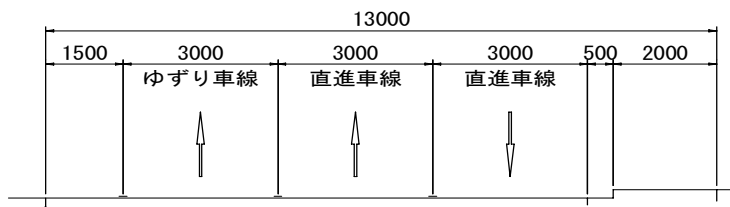
【横断面図】
