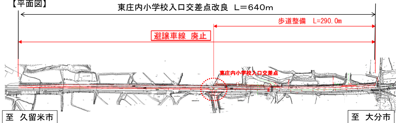
【平面図】
