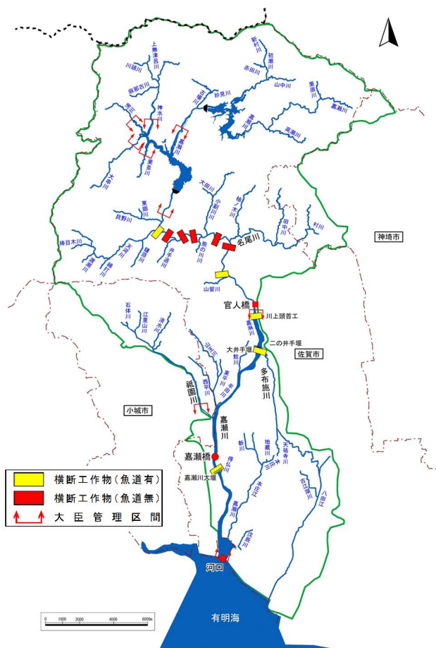
図 2.3.2 横断工作物位置図
