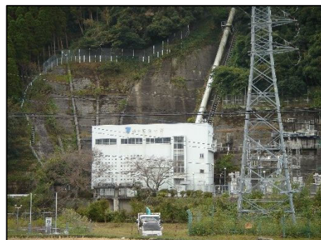
写真 2.2.5 鮎の瀬発電所
