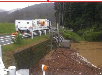
笠掛樋門
