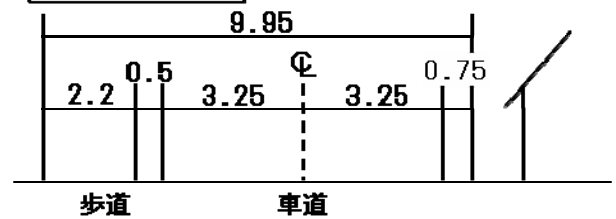
横断面 (整備前)
