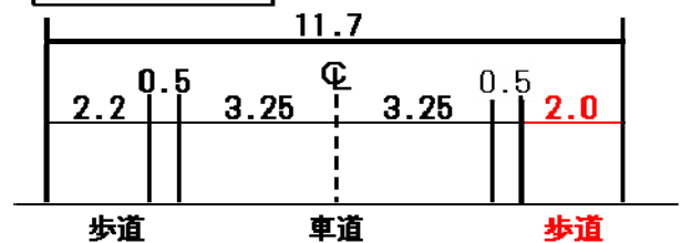
横断面 (整備後)
