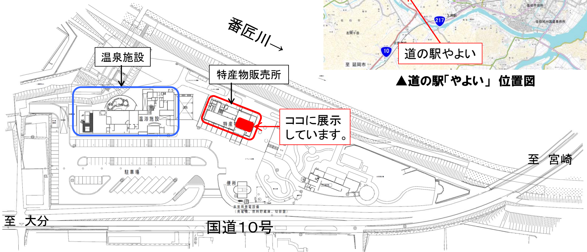
▲道の駅「やよい」平面図
