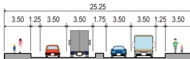
▲ 標準断面図
