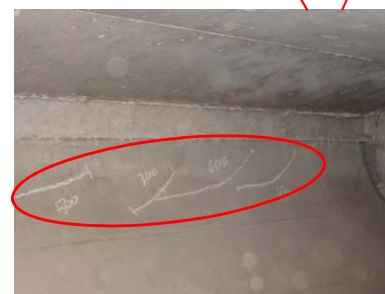
箱桁内面側のひび割れ
