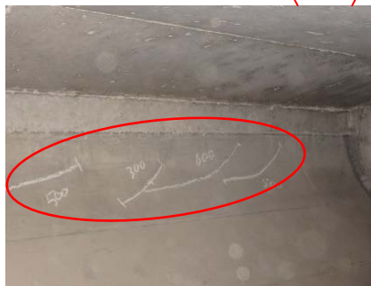
【箱桁内面側のひび割れ】
