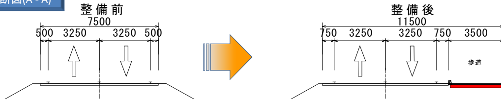
横断面(A-A)
