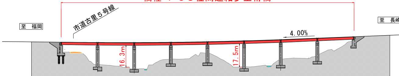
側 面 図
