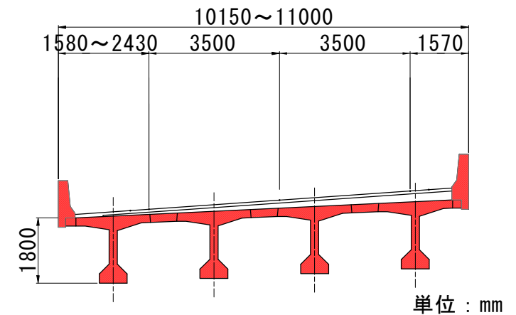
標準断面図
