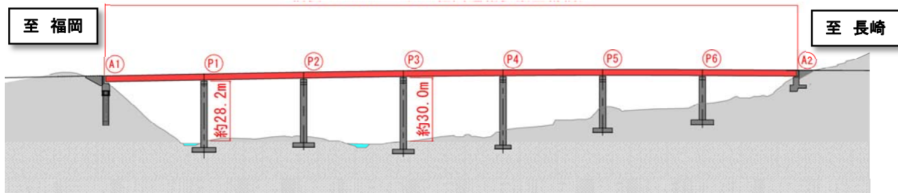
橋長 L=320m (PC7径間連結T桁橋)
