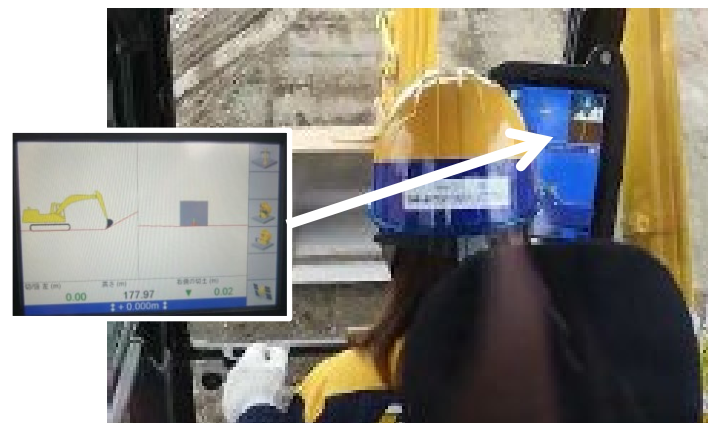
▲作業は運転席モニタを確認
