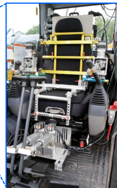
簡易遠隔操縦装置（ロボQS）
