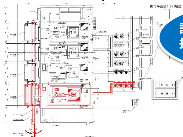
ポンプ設備据付（1F）平面図
